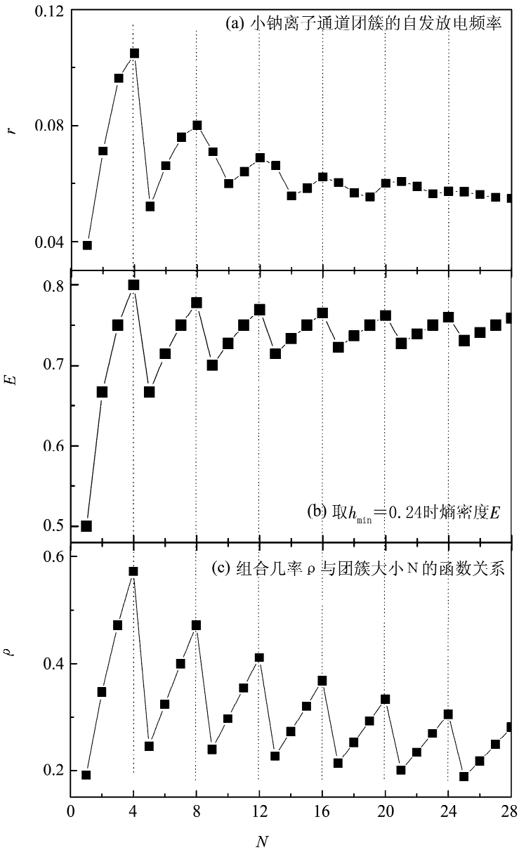
图 4-3-4 放电频率、熵密度和组合几率的关系
