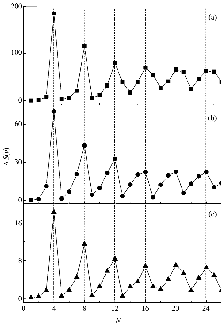
图 4-3-8 从 N=1\sim 26 变化时,系统的信号编码能力 \Delta S(v) 曲线
