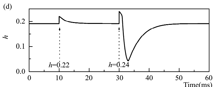
图 4-3-1 膜电位动力学
