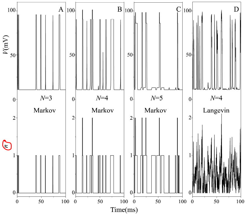
图 4-3-2 动作电位的随机系列和相应的开放通道数
