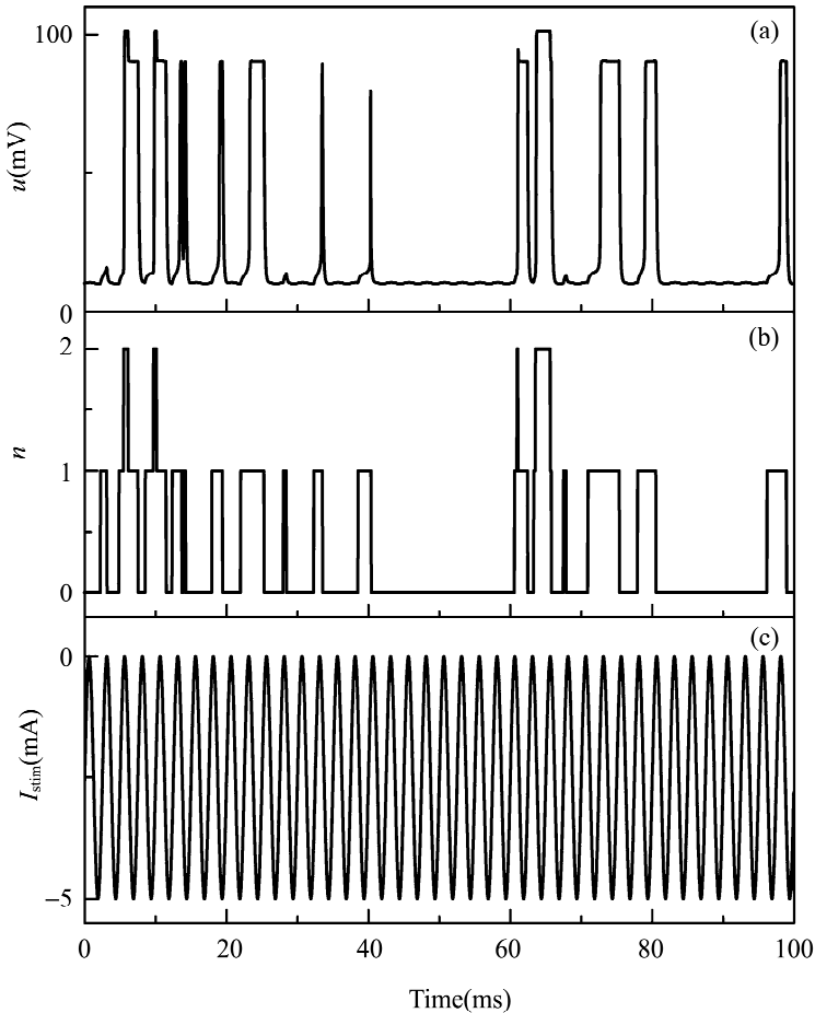
图 4-3-5 系统对外界周期信号的反应
