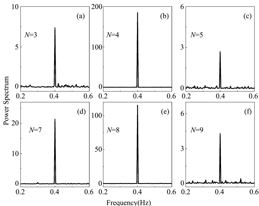
图 4-3-6 加有周期电流的系统的功率谱
